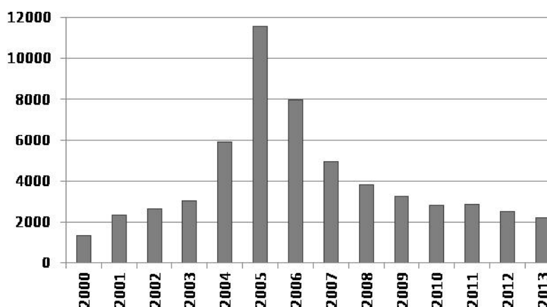
Rysunek 1. Liczba orzeczonych separacji w Polsce
