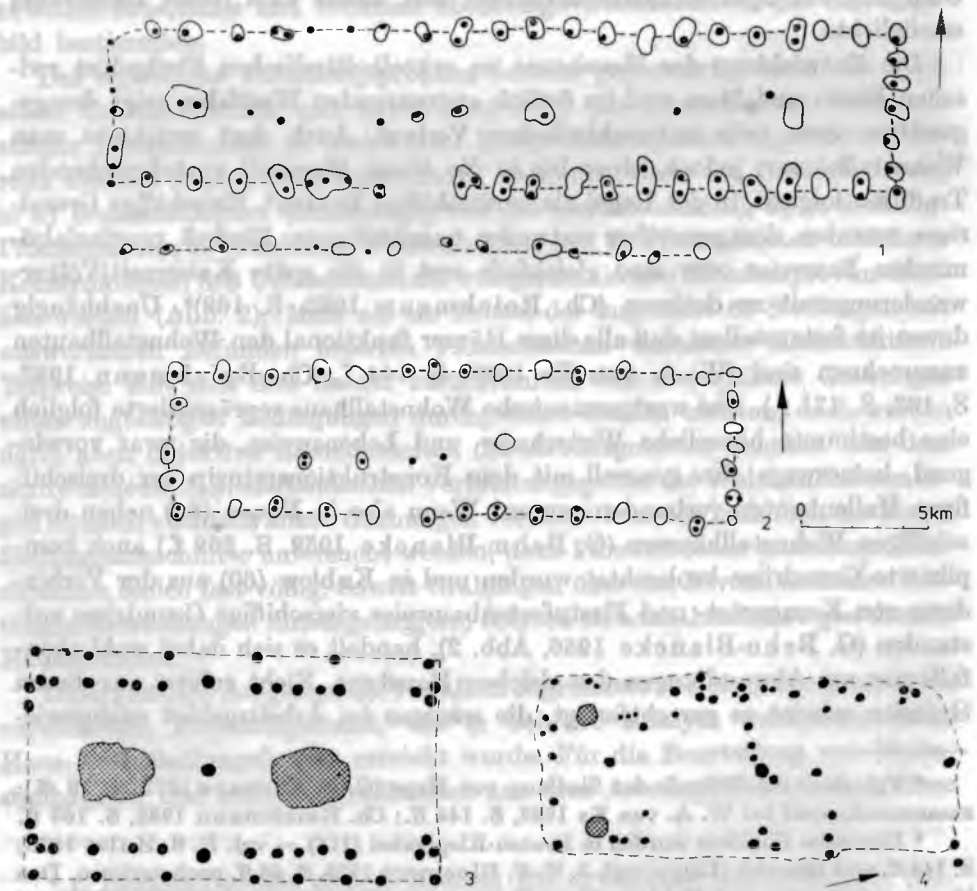
Abb. 4. Große, langrechteckige Pfostenhäuser: 1. - 2. Tornow (65), Haus 23 und Haus 49; 3. Wólka Łasiecka (47), Haus 3; 4. Tokarnia (43), Haus 1
