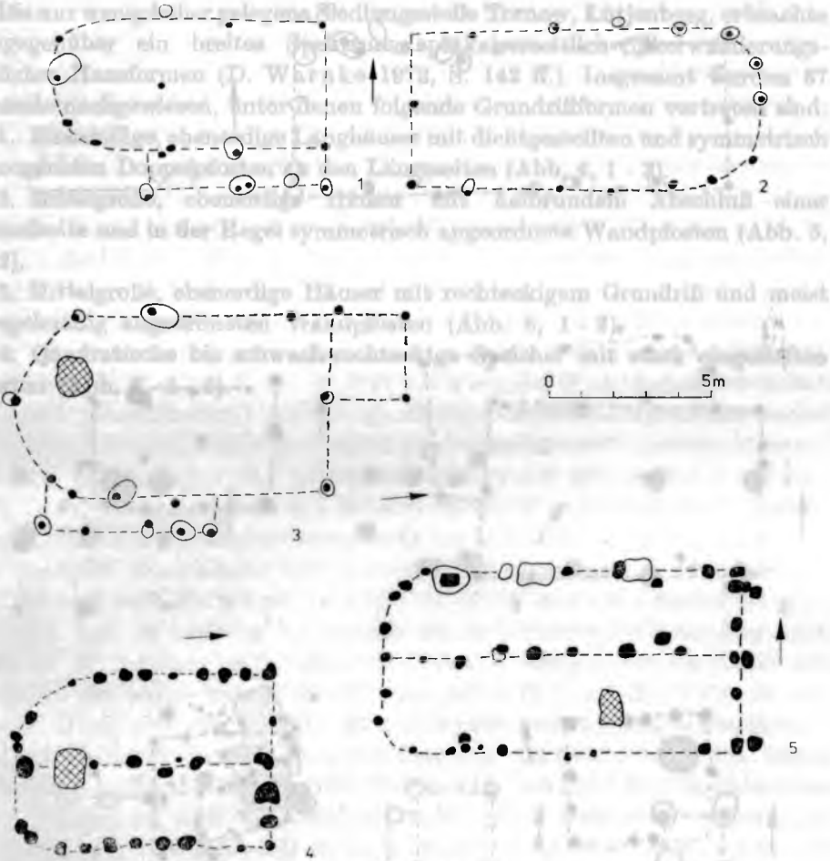
Abb. 5. Mittelgroße Pfostenhäuser mit halbrundem Abschluß: 1. - 3. Tornow (65), Haus 20, 74 und 138; 4. Frankfurt-Kliestow (56), Haus 2; 5. Langewahl (63), Haus 3
