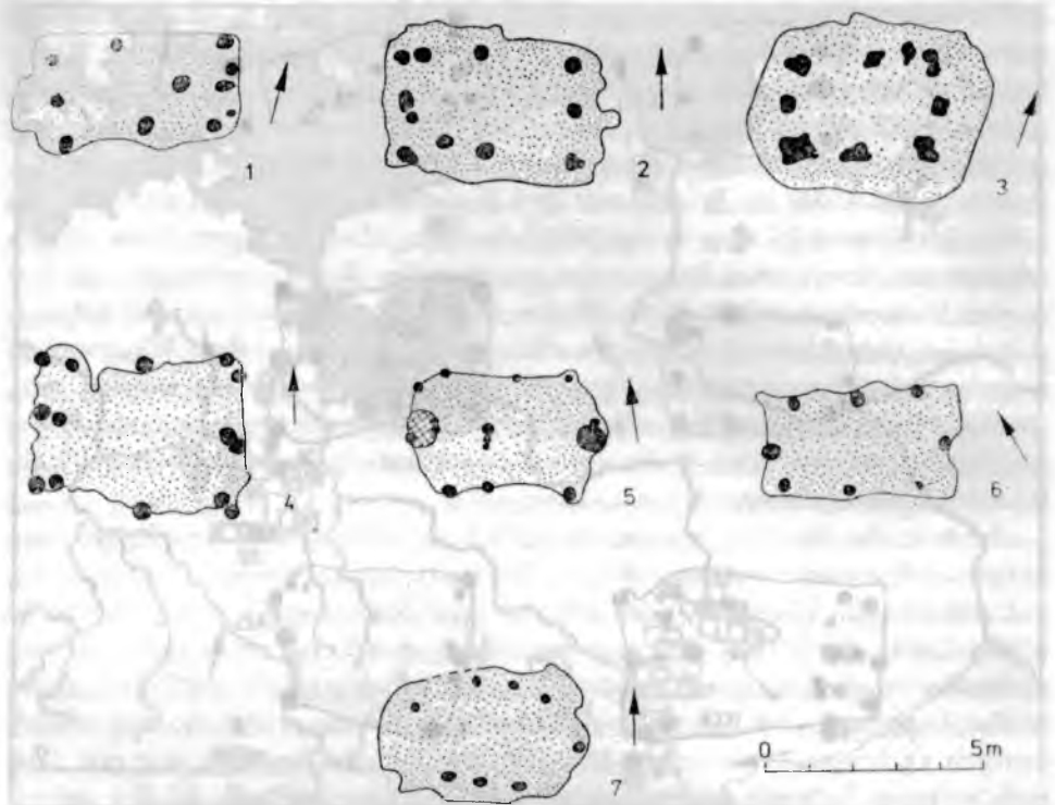
Abb. 10. Grubenhäuser der Form C 2: 1. Chorula (4), Haus 1; 2. - 3. Gröben (57), Haus 4 und 7; 4. Zarzyca (49) Grubenhäuser der Form D 2: 5. Frankfurt-Kliestow (56), Haus 7; 6. Klein Köris (61), Haus 7; 7. Wüste Kunersdorf (67), Haus 5
