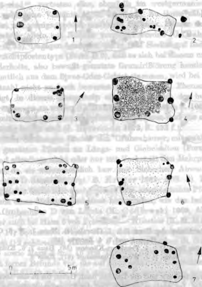
Abb. 9. Grubenhäuser der Form C: 1. Byhleguhre (51), Haus 1; 2. Chorula (4), Haus 2; 3. Danków (6), Haus 400; 4. Kościeliska (12), Haus 1; 5. Ligota (19), Haus D; 6. Mierzyce (22); 7. Opatów (28), Haus 1
