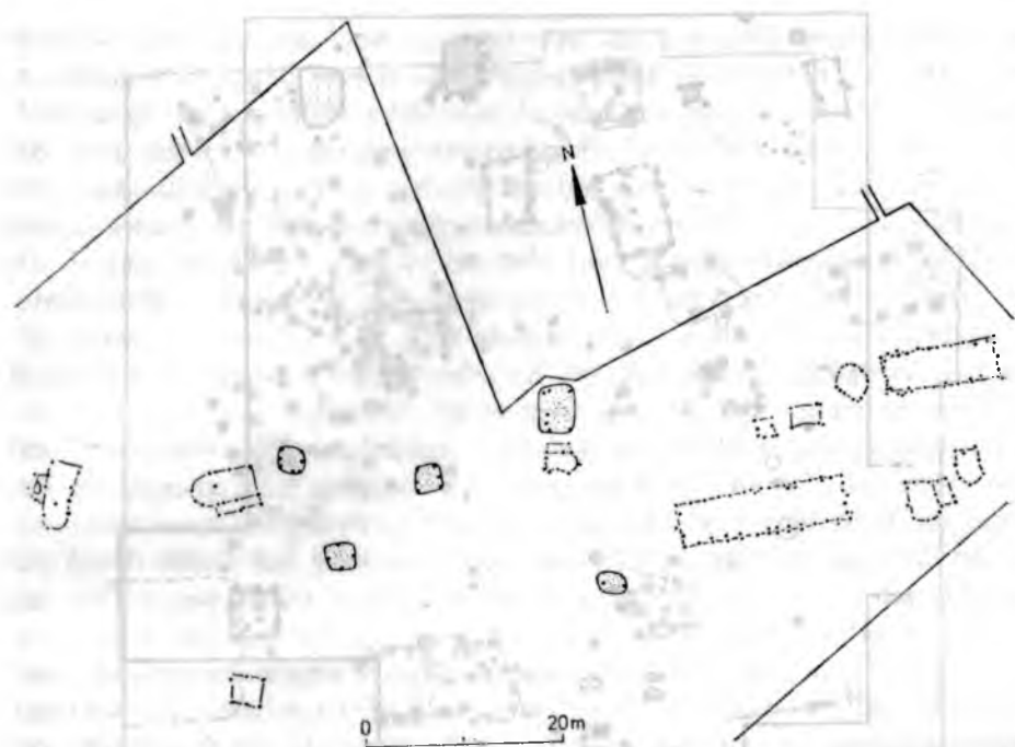
Abb. 12. Tornow (65), Lütjenberg, Siedlungskomplex — wahrscheinlicher Plan eines Bauhorizontes
