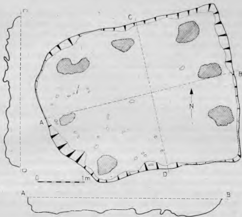
Abb. 15. Dessau-Mosigkau. Grundriss des Grubenhauses 10 (Häuser- ring 1). Nach B. Krüger 1967
