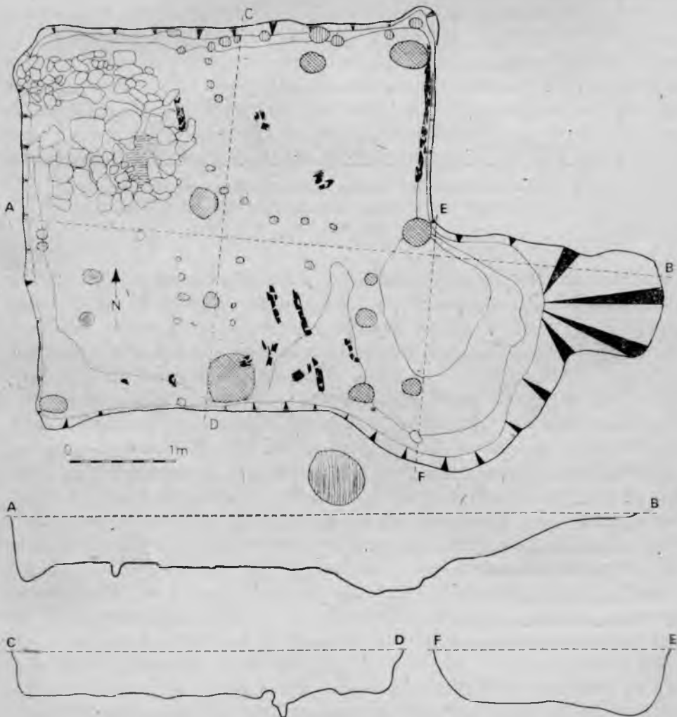
Abb. 4. Dessau-Mosigkau. Grundriss des Grubenhauses 19 (Häusering 4). Nach B. Krüger 1967
