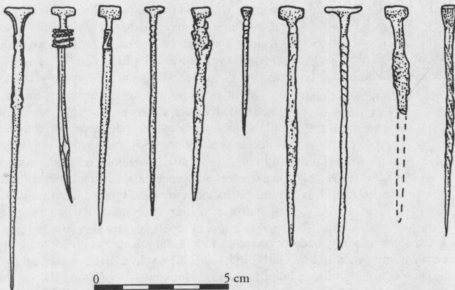
Ryc. 10. Stylusy z Ostrowa Tumskiego w Poznaniu (rys. O. Antowska-Gorączniak)
