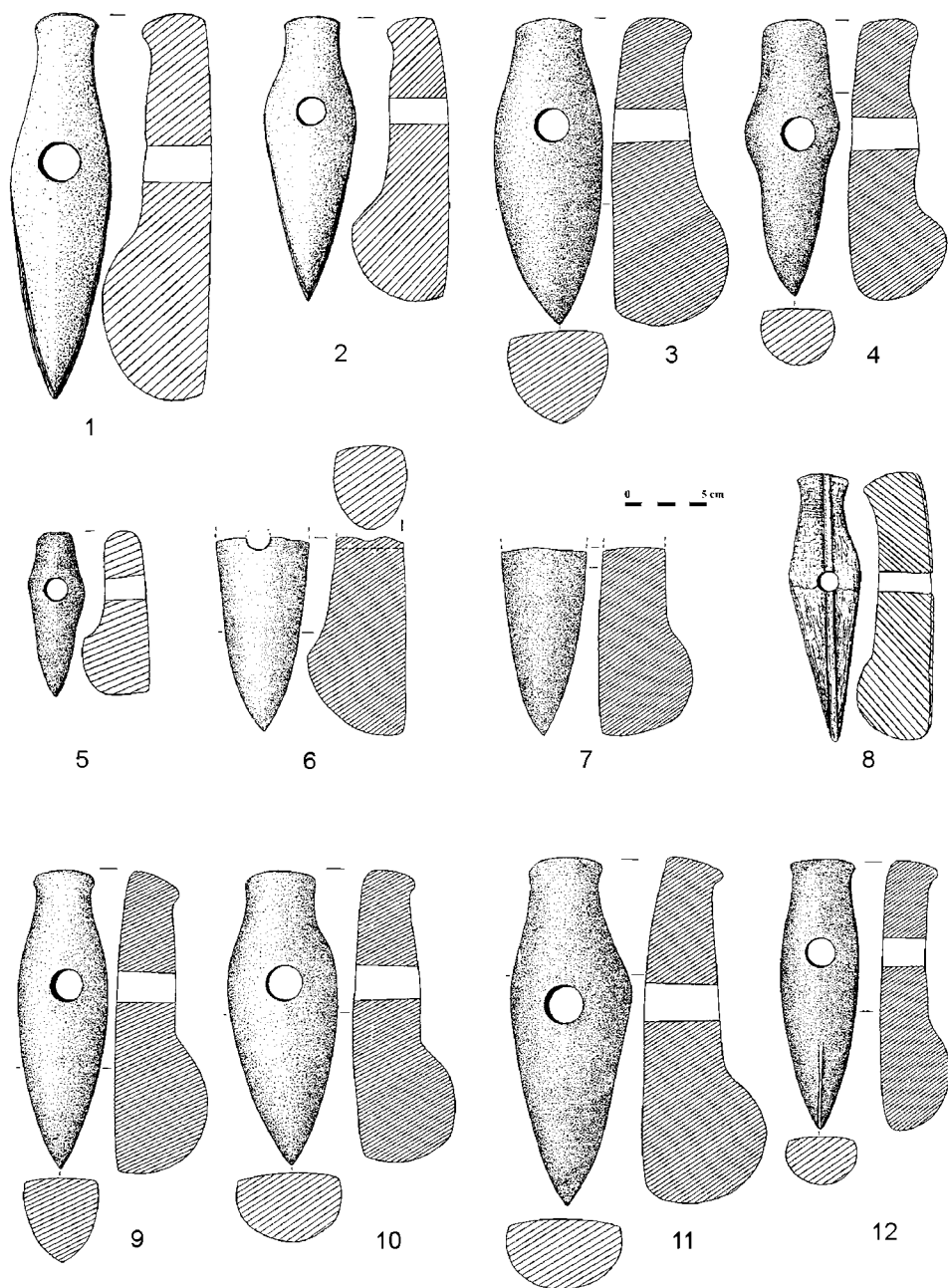
Fig. 2. Examples of 'spade-like' axes of west Volhynia and Podolia: 1. Narodyš, 2. Kornič, 3. Dašava, 4. Zabučia, 5. Targovica, 6, 7. Demidovka, 8. Dzinogrod, 9. Griadki, 10. Halič, 11. Černylava, 12. Bohorodčany (sketches by V. Konopla)
